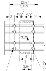
ELEVATION
