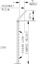
END ELEVATION
