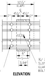
ELEVATION
