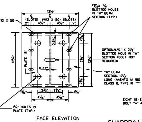
FACE ELEVATION
