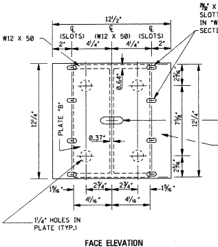
FACE ELEVATION
