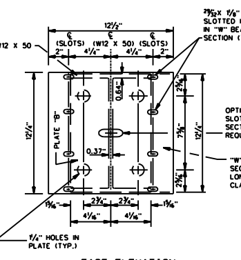
FACE ELEVATION
