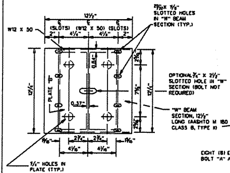
FACE ELEVATION
