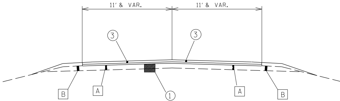
TYPICAL FOR SR 371 STA. 48+00 - EOP STA. 283+82
