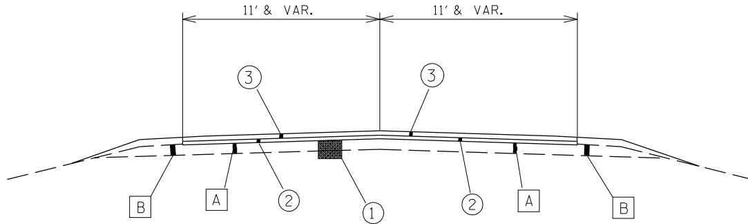
TYPICAL FOR SR 371 BOP STA. 5+00 - STA. 48+00
