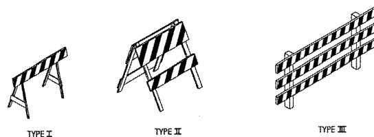
STANDARD BARRICADES
