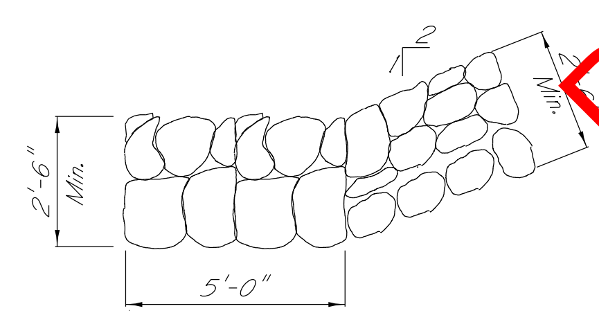
RIPRAP APRON DETAILS
