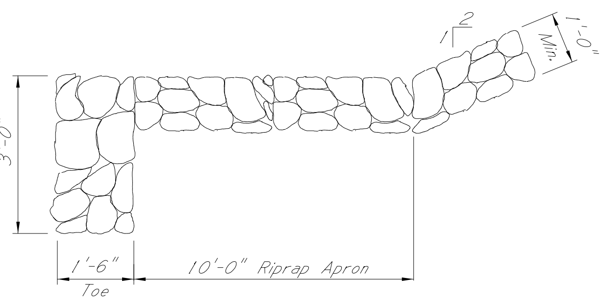
RIPRAP APRON & TOE DETAILS (Not to scale)
